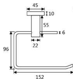
Toilet roller holder
